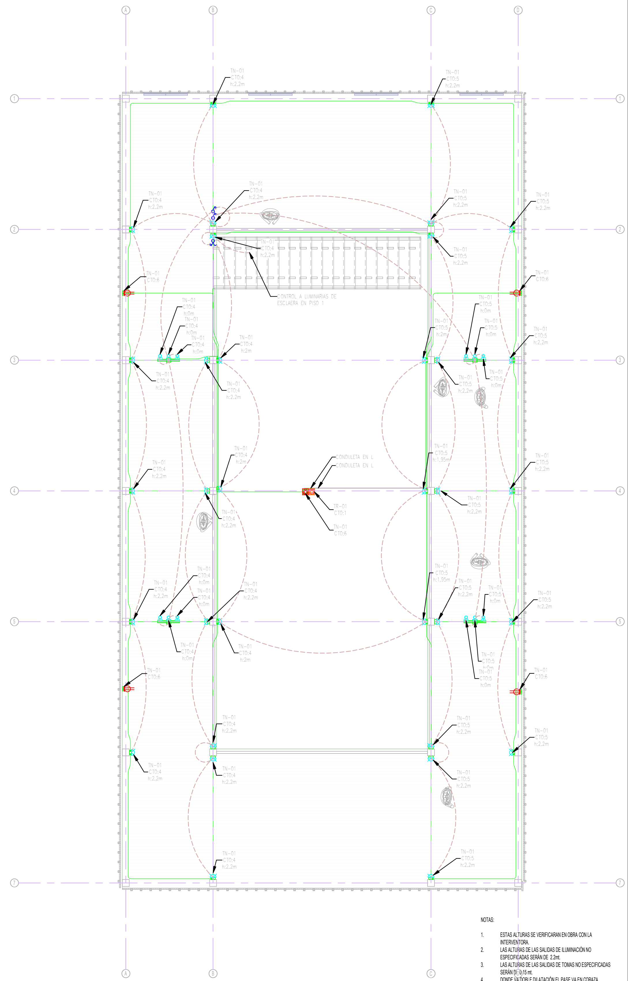
2 ELE - TOMAS - ILUMINACIÓN - SEGUNDO PISO 1:50
