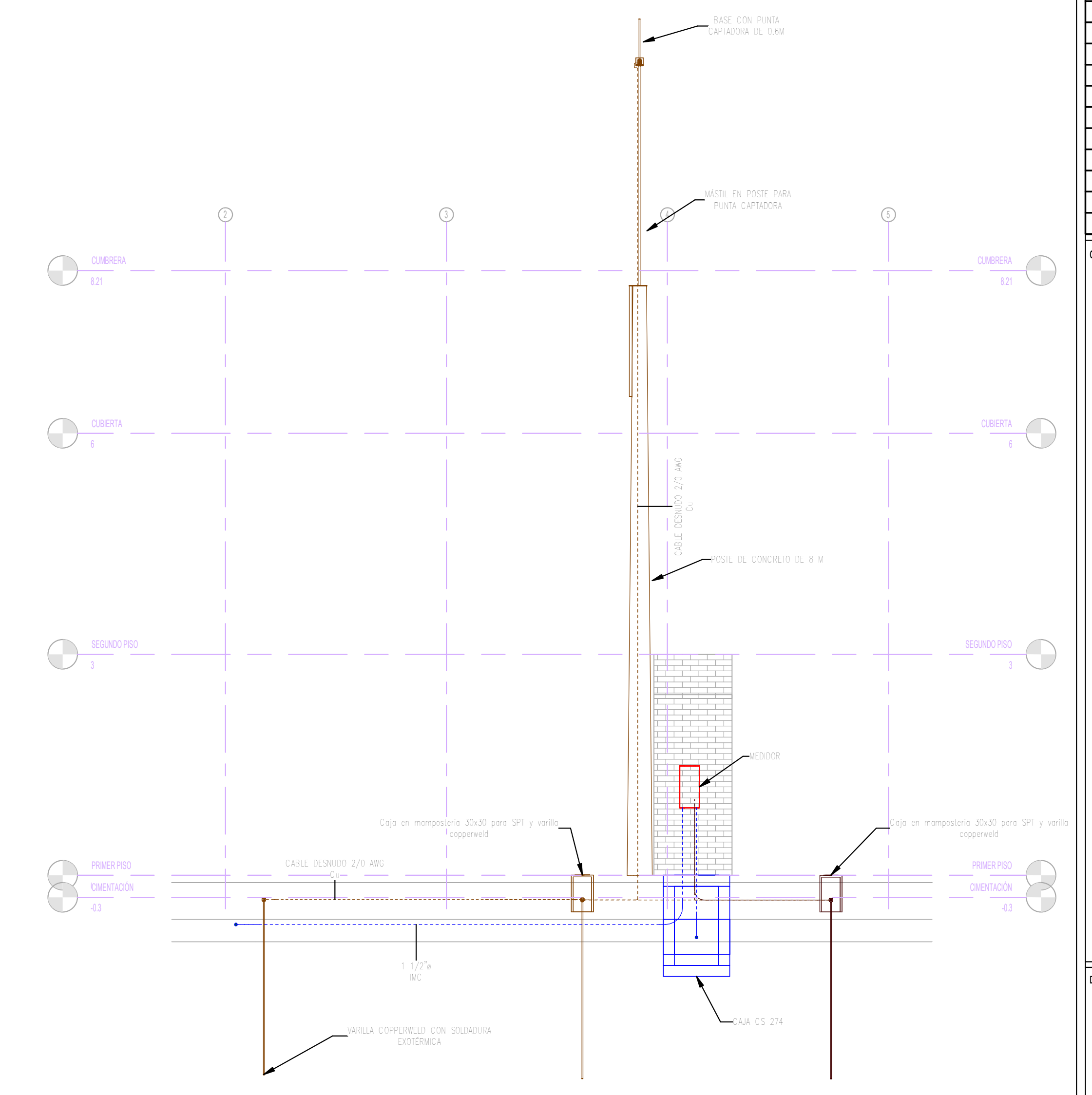
1 MEDIDOR ELÉCTRICO 1:50
