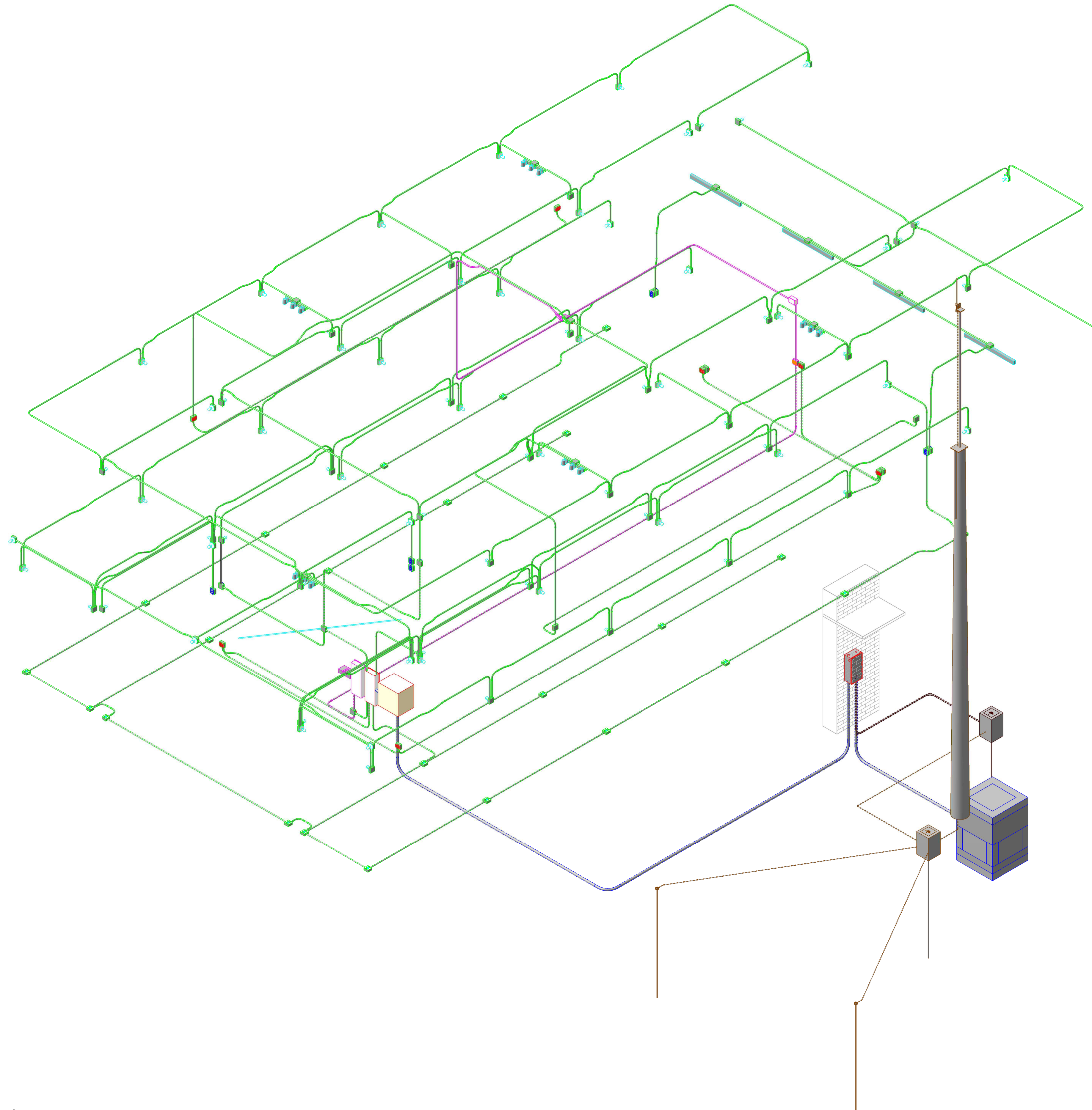
1 ISOMÉTRICO
